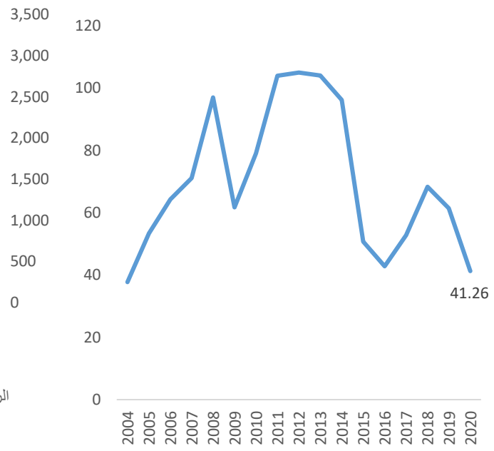
رسم بياني 1-3: متوسط سعر النفط BRENT
