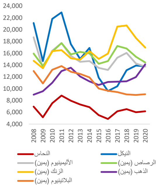
رسم بياني 1-4: أسعار المعادن
